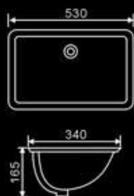
DB-540E Size: 530x340x165 mm
